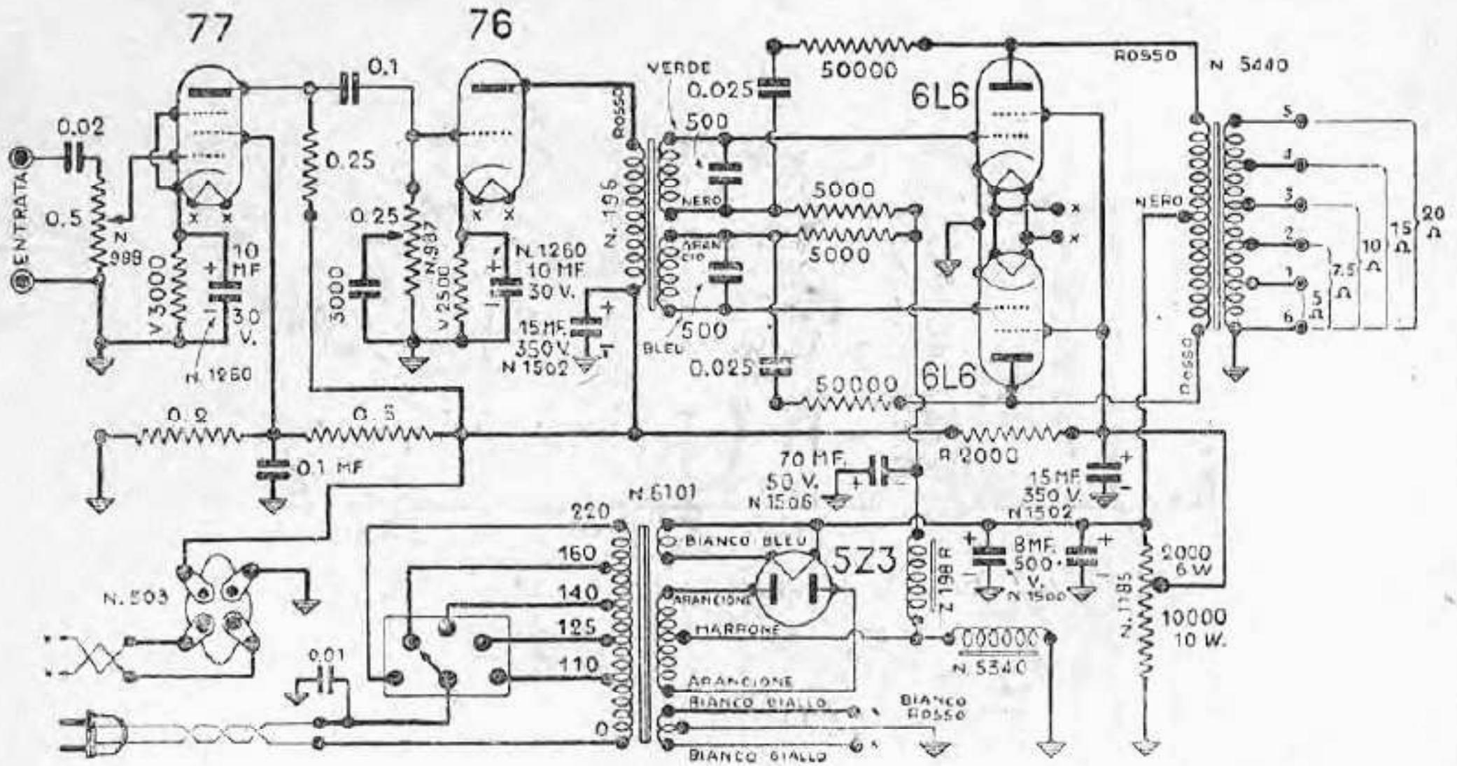
AMPLIFICATORE G. 27
