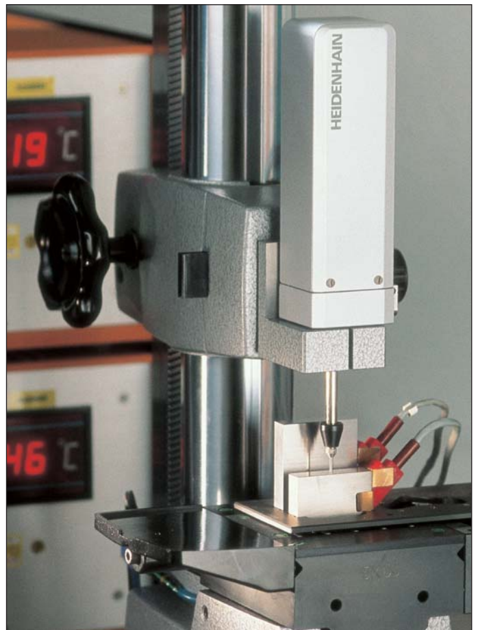
Calibration de cales-étalon
