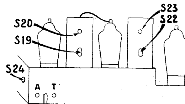
Disposition des noyaux ajustables des transformateurs M.F. et de celui du filtre d'antenne (S24).
